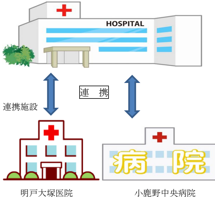
図 1：研修体制
